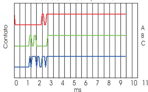
Ajustando disjuntor para atender aos requisitos de tempo
